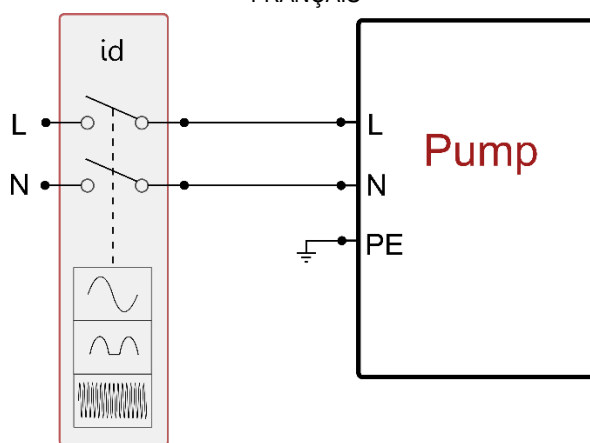
Exemple d'installation
