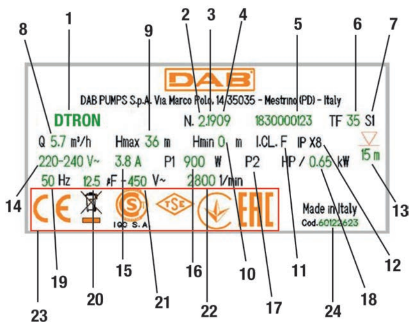
Eticheta tehnică
