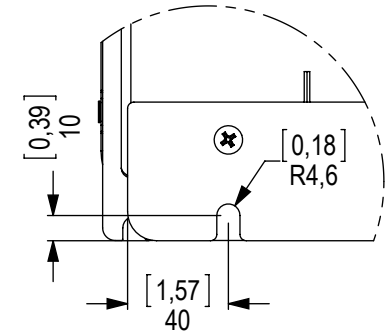
DETALHE B ESCALA 1 : 3
